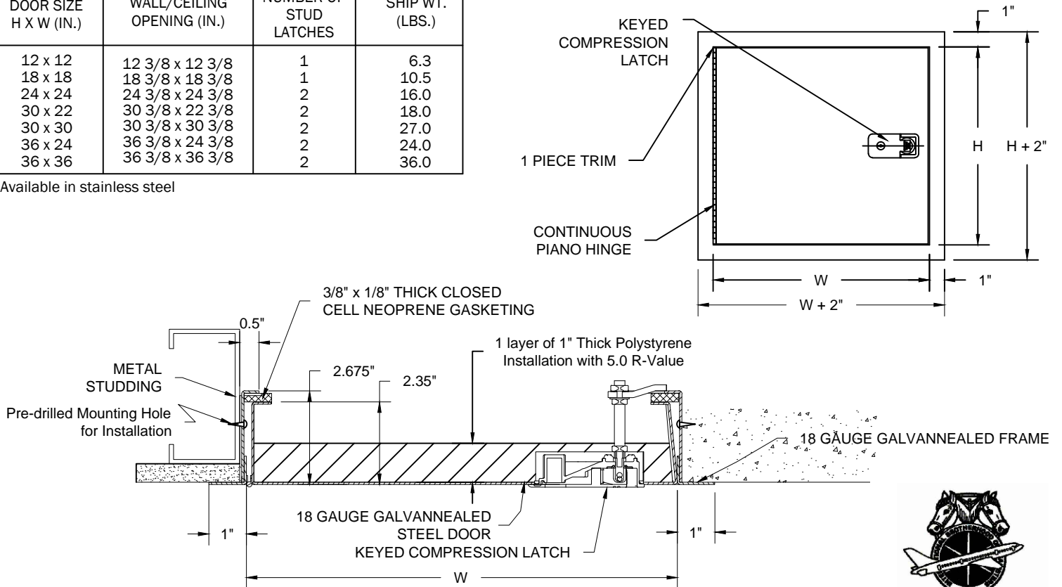
SECTION A-A
