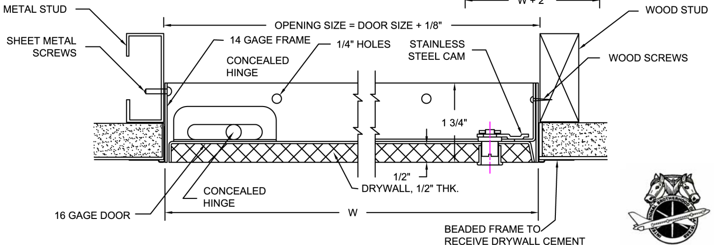
SECTION A-A
